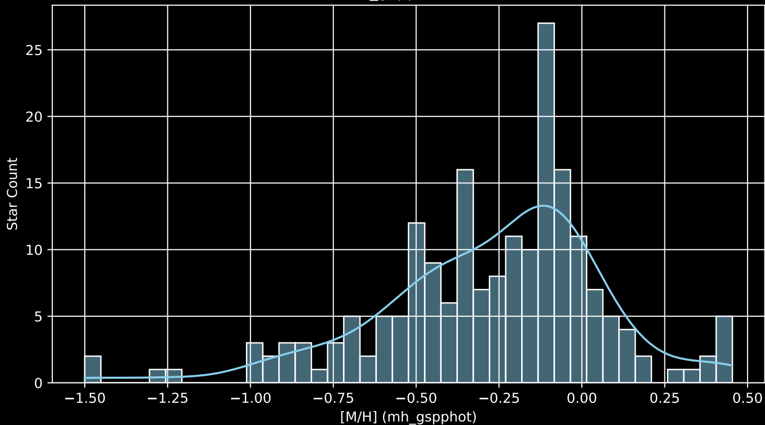
APOGEE DR17 Field: [283-38-O_TESS [M/H] (mh_gspphot) (n= 196)
