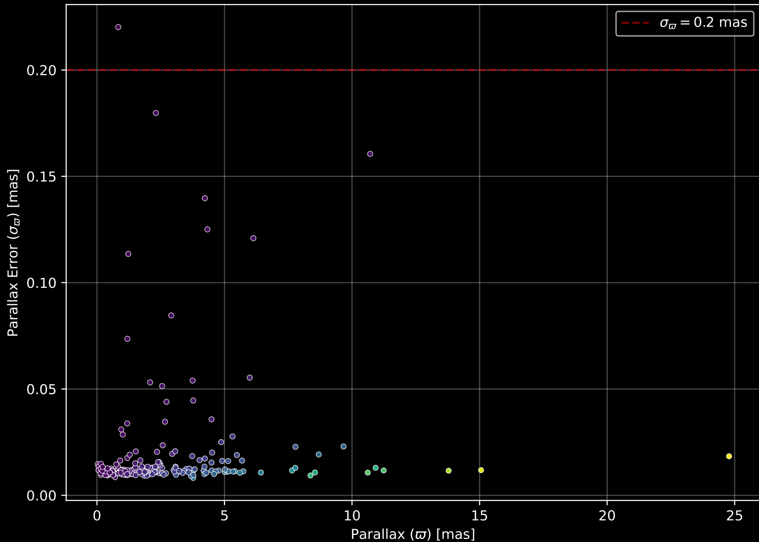
APOGEE DR17 Field: [283-38-O_TESS] Parallax Quality (n= 196)
