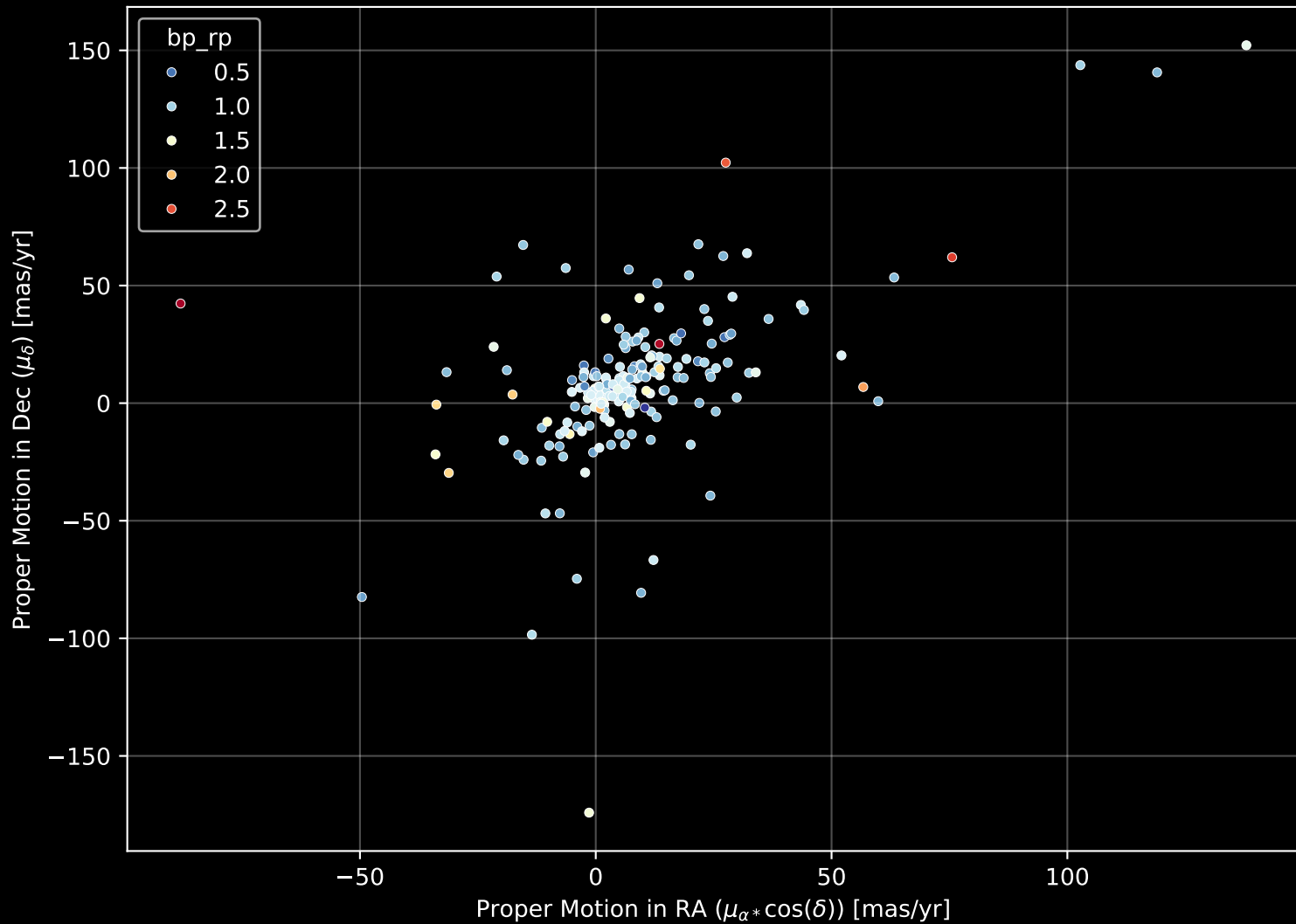
APOGEE DR17 Field: [283-38-O_TESS] Proper Motion Diagram (n= 196)
